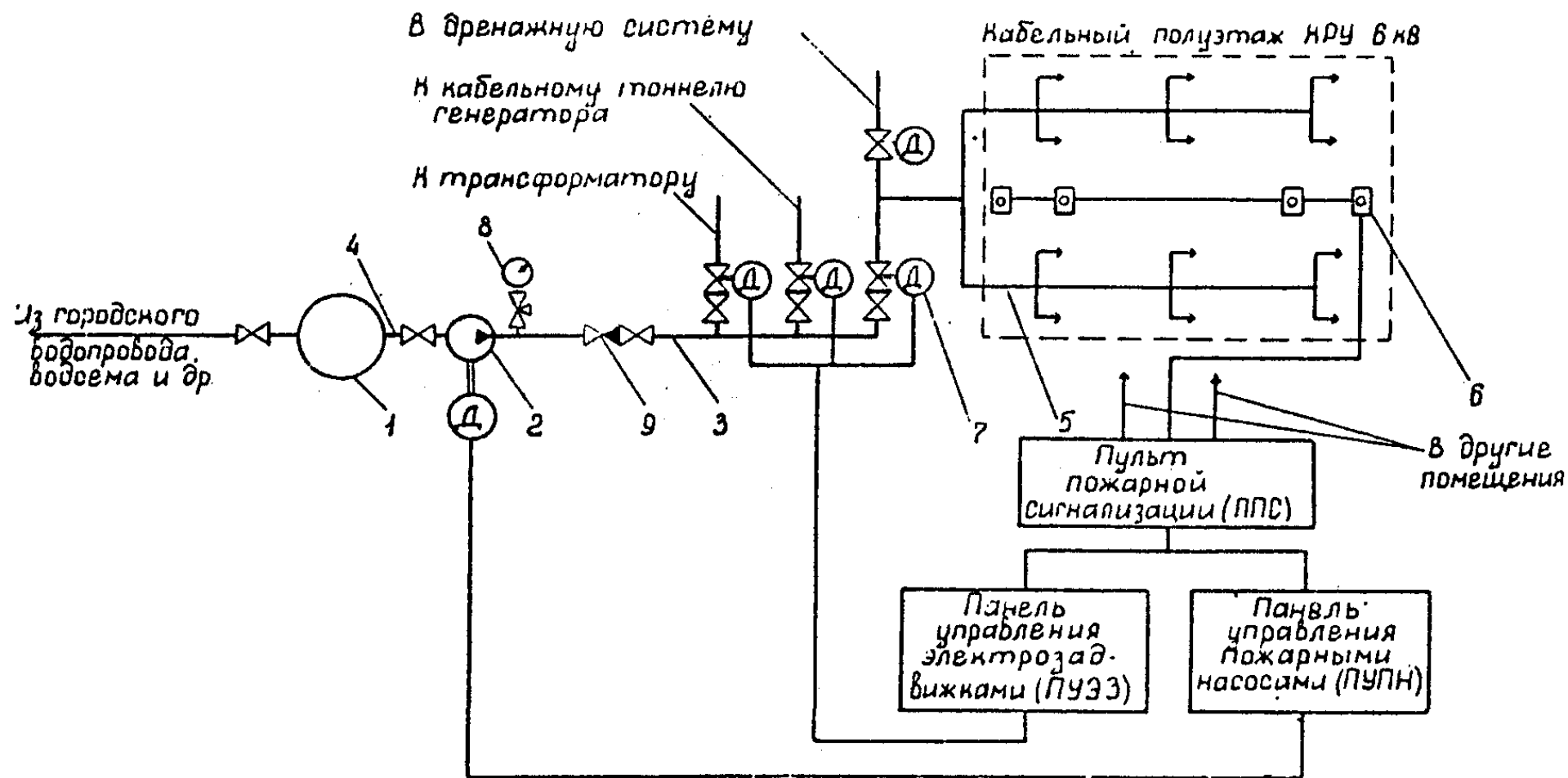
Принципиальная схема установки водяного пожаротушения:
